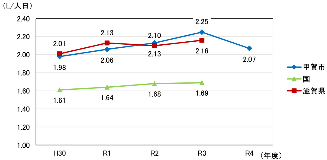
図4-1-6 浄化槽汚泥の1人1日平均排出量の推移
