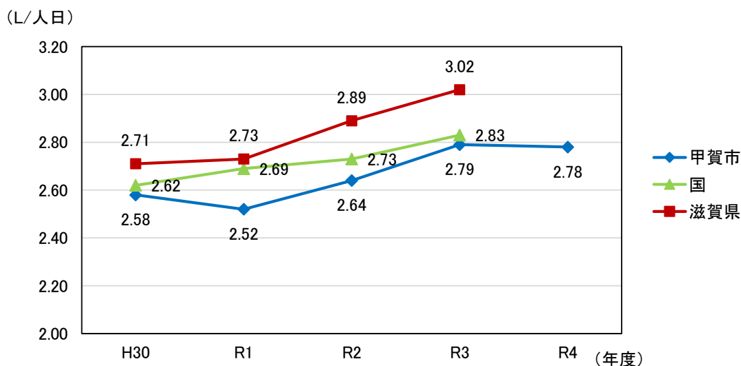
図4-1-5 し尿の1人1日平均排出量の推移
