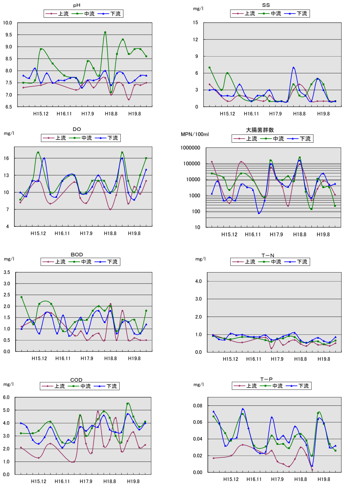
図 24 杣川経年推移
