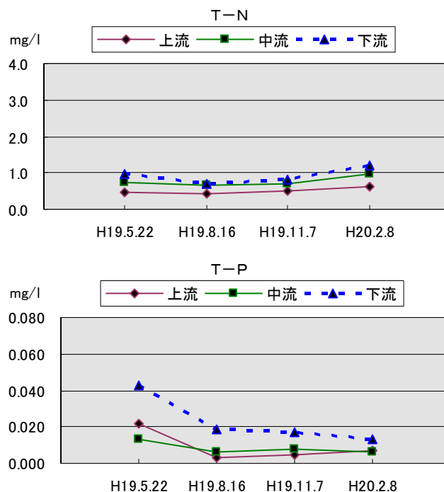
図 8 T-N・T-P 結果
