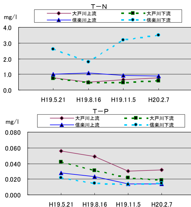
図 18 T-N・T-P 結果
