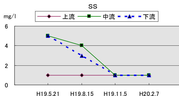
図 11 COD・SS結果
