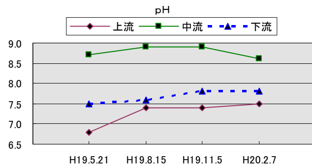
図 9 流量・pH 結果
