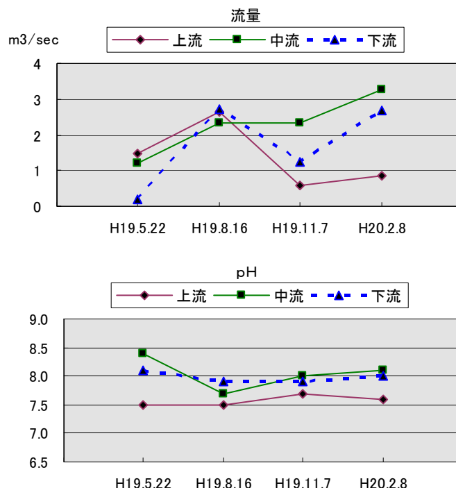
図 4 流量・pH 結果
