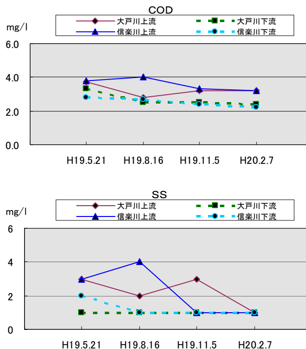
図 16 COD・SS 結果
