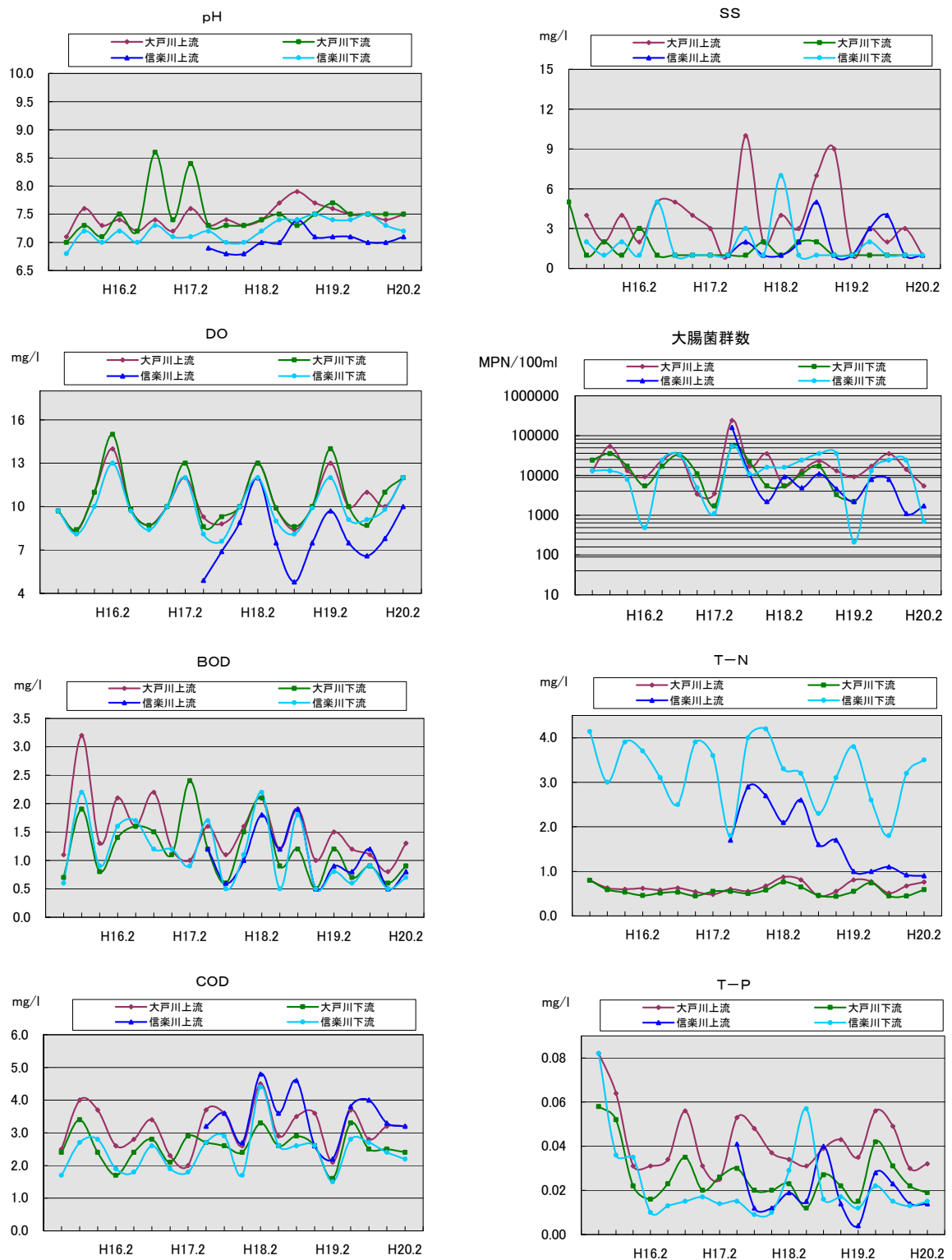
図 25 大戸川・信楽川経年推移
