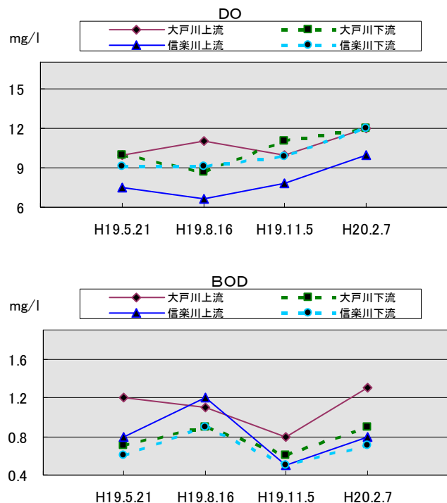
図 15 DO・BOD結果
