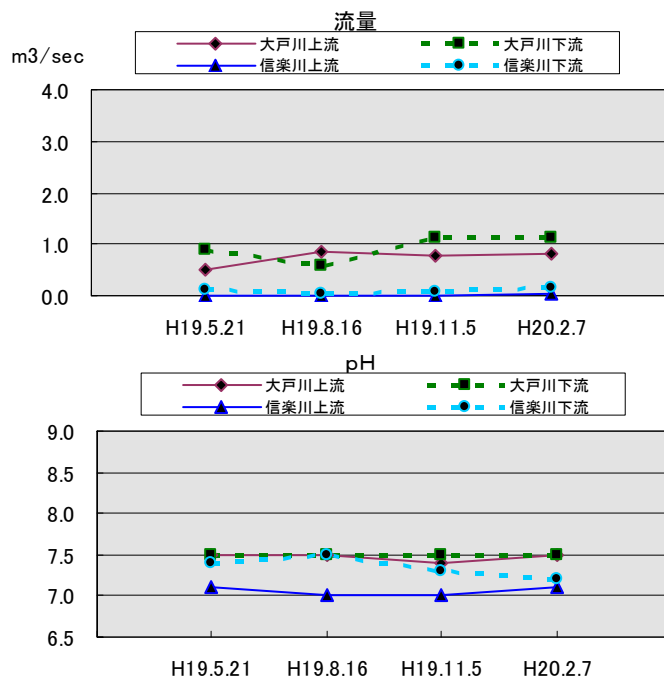
図 14 流量・pH結果
