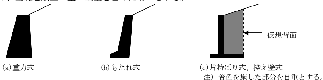
図12-4 擁壁の自重
