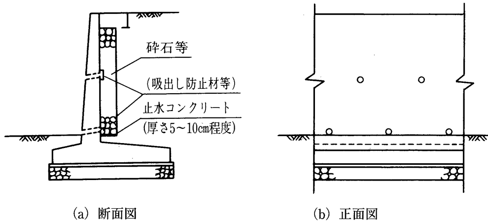
図 12-14 水抜穴の配置図
