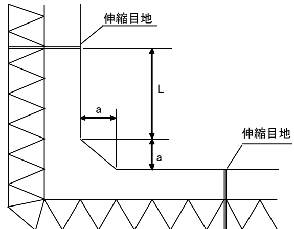
(b) 平面図
