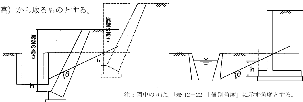
図 12-20 水路、河川に接している場合の根入れ深さ
