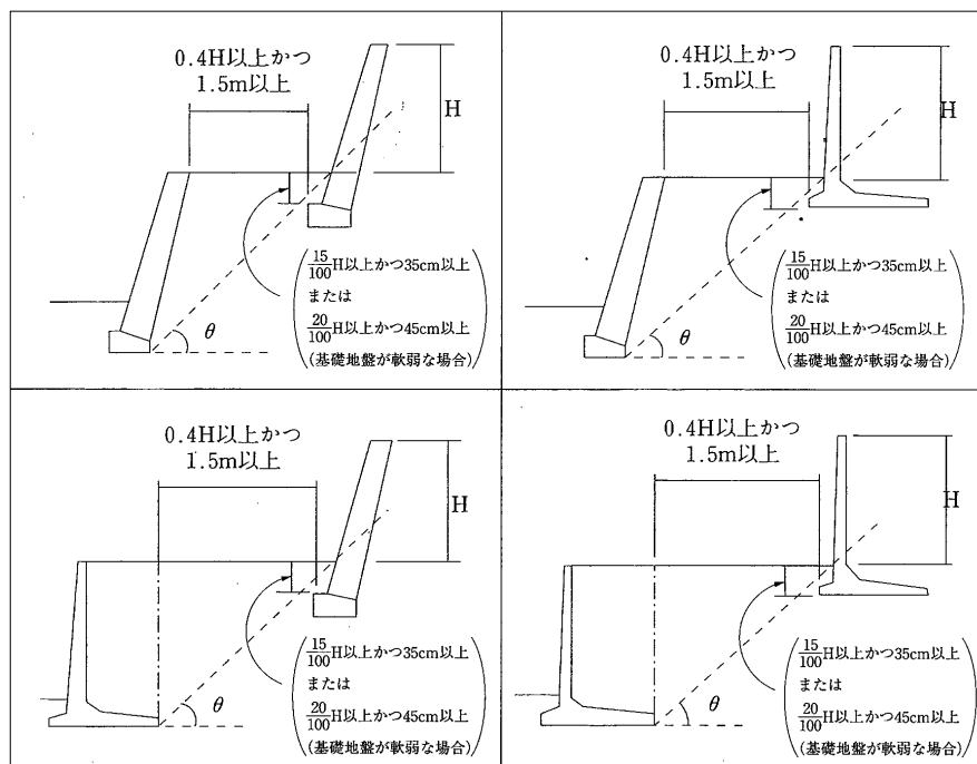
図12-22 上部・下部擁壁を近接して設置する場合
