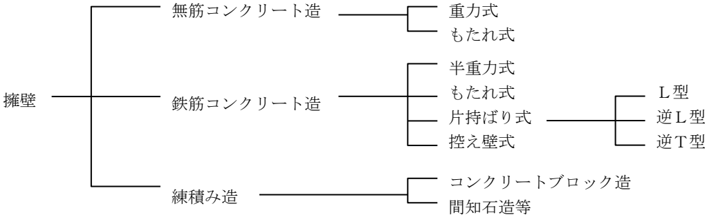
図12-3 擁壁の種類
