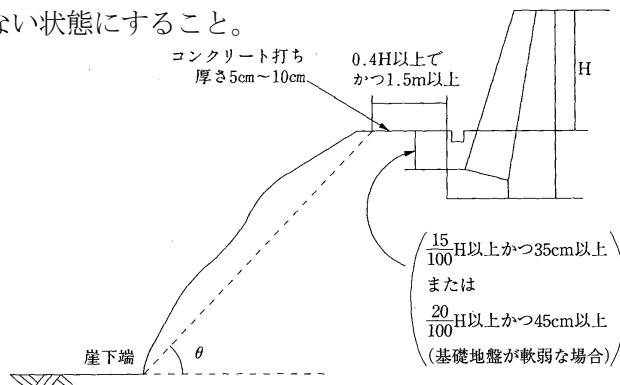
図12-21 斜面上に擁壁を設置する場合
