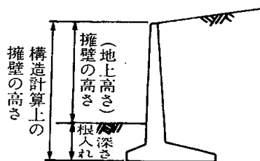
図12-7 擁壁の高さの考え方
