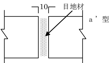
図12-16 伸縮目地
