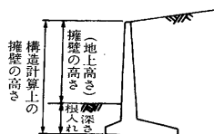
図12-2 擁壁の高さの考え方
