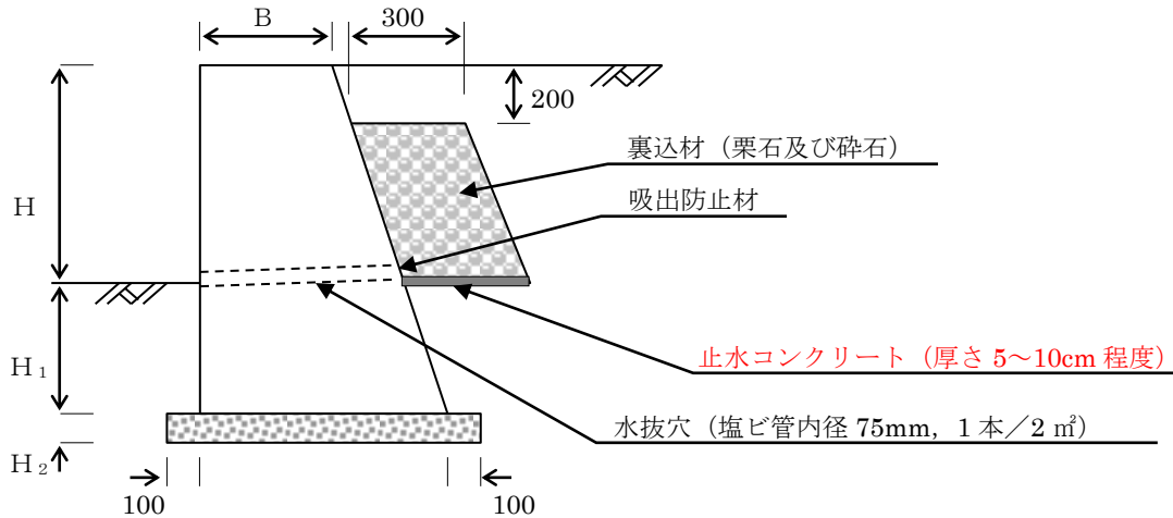
図12-12 重力式擁壁標準図
