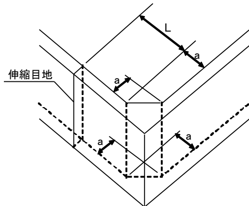
(a) 立体図
