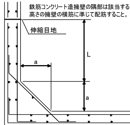
(b) 平面図
