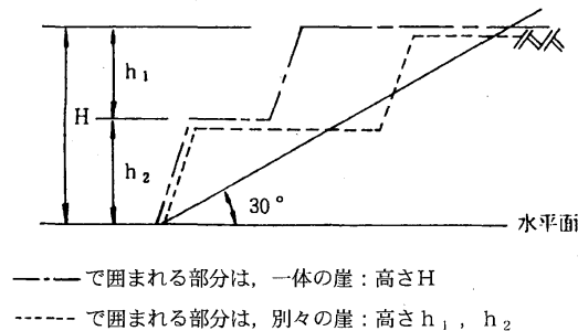
図12-1 一体のがけ、別々のがけ
