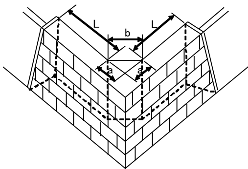
(a) 立体図
