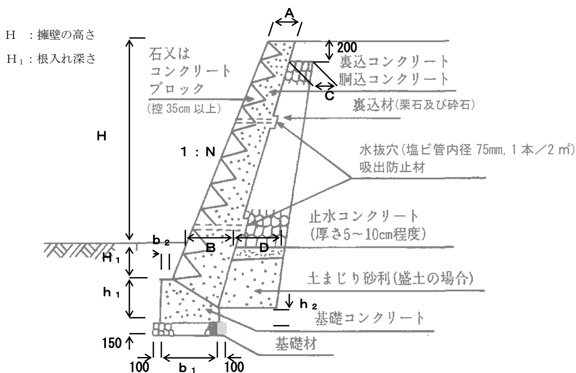
図12-11 練積み造擁壁の構造
