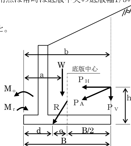
図12-8 合力作用位置の求め方
