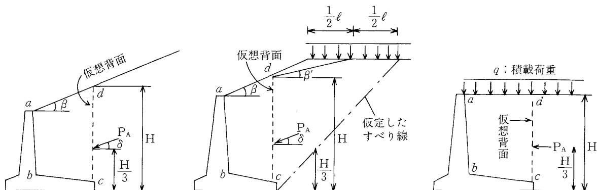
(a) 地表面が長大斜面の場合
