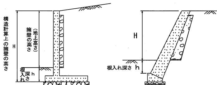
図 12-18 擁壁の根入れ深さ
