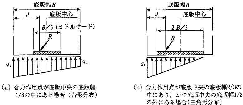
図12-9 地盤反力度の求め方
