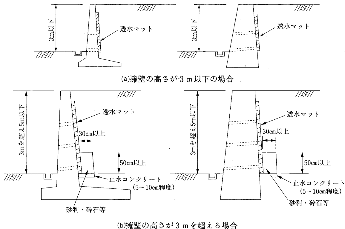
図12-15 透水マットの取付け断面
