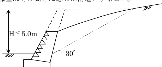
図12-10 盛土部で背後に斜面がある場合の擁壁高さ
