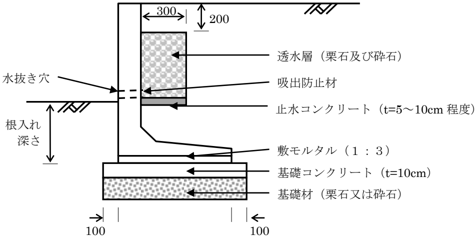
図12-13 プレキャスト擁壁標準断面図
