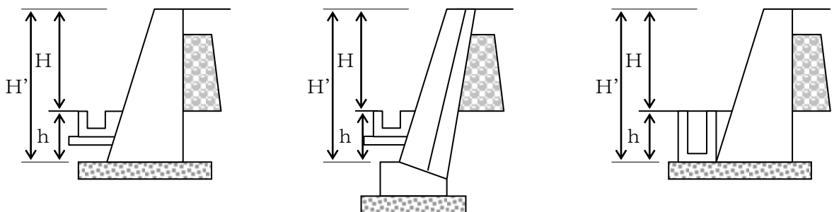
図 12-19 擁壁前面に排水構造物を設ける場合の根入れ深さ
