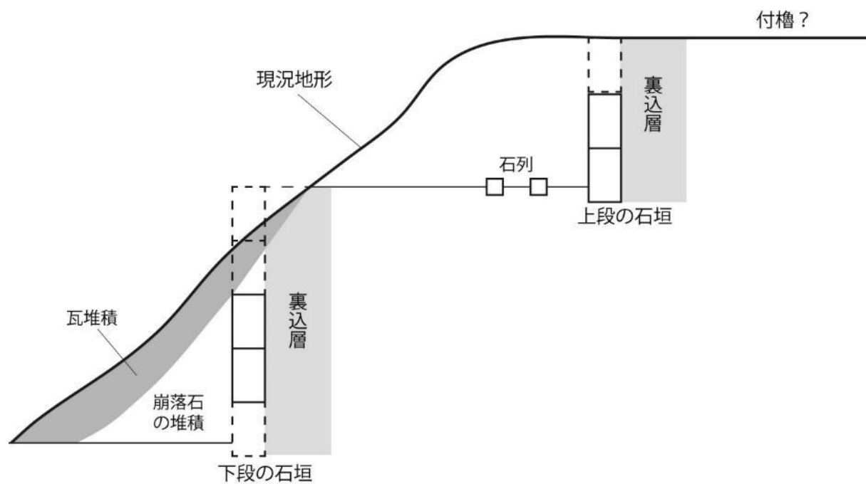
図7 東櫓台周辺の上下2段の石垣模式図
