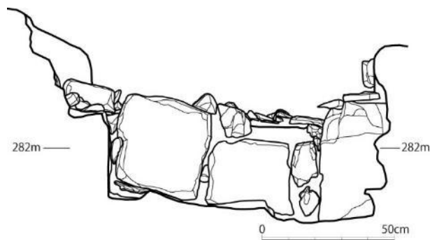
図5 東櫓台の石垣(上段)立面図② 1:20
