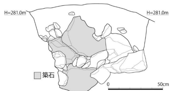
図6 下段の石垣立面図 1:20
