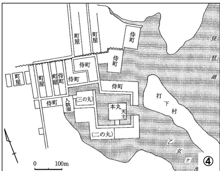
図版 1 ①位置図 ②・③地形測量図 ④大溝城模式図 ⑤寛文四年頃の本丸 (⑦より)
