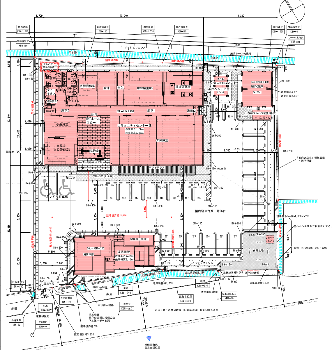
配置図 1/200
