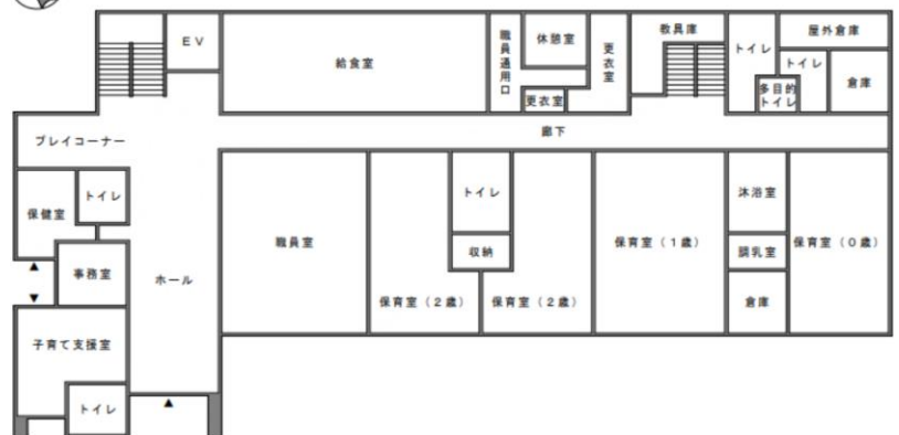
■ 1 階 平面 図
