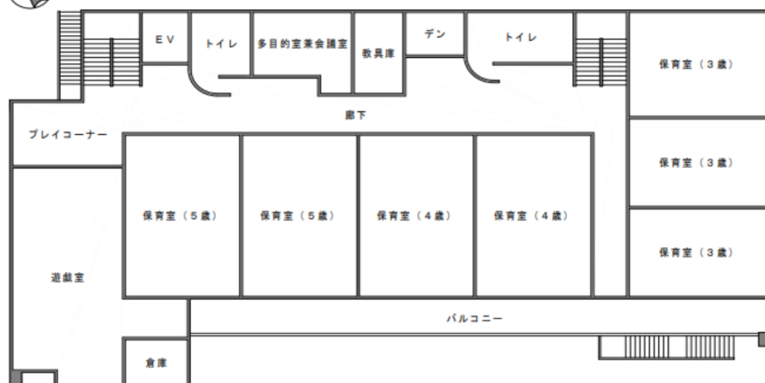
【2F 平面図】
